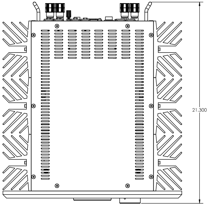
SCALE 1 : 3
